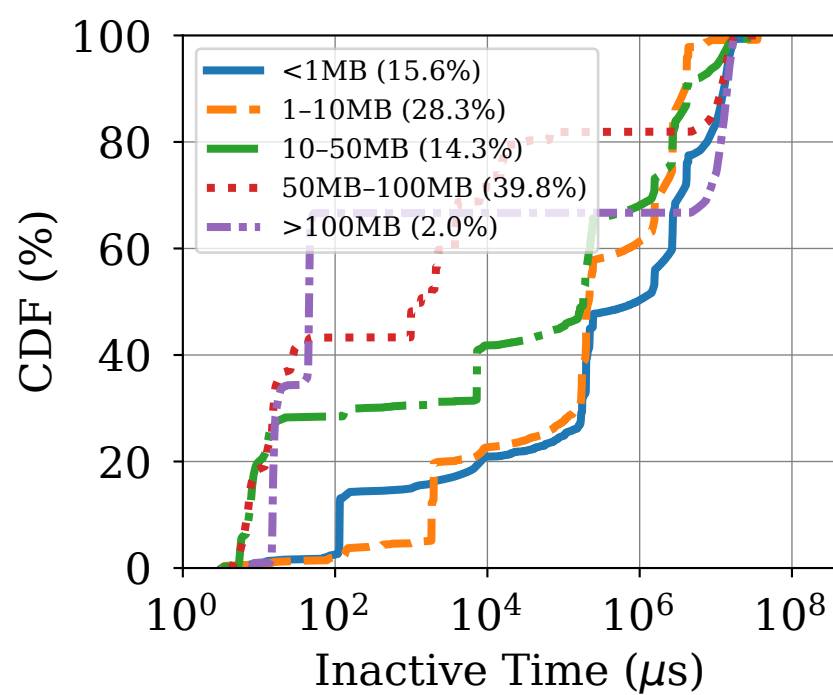
(d) T5-11B
