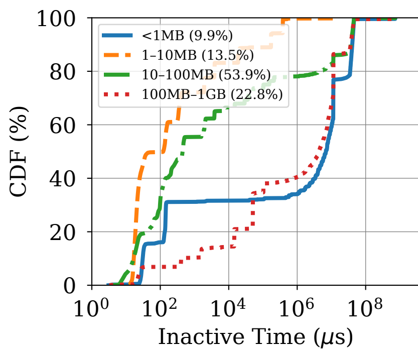
(c) Llama3-70B
