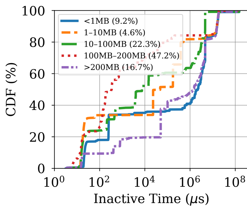
(a) Llama3-8B
