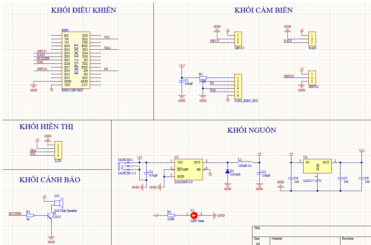
Hình 2.2 Sơ đồ nguyên lý của hệ thống
