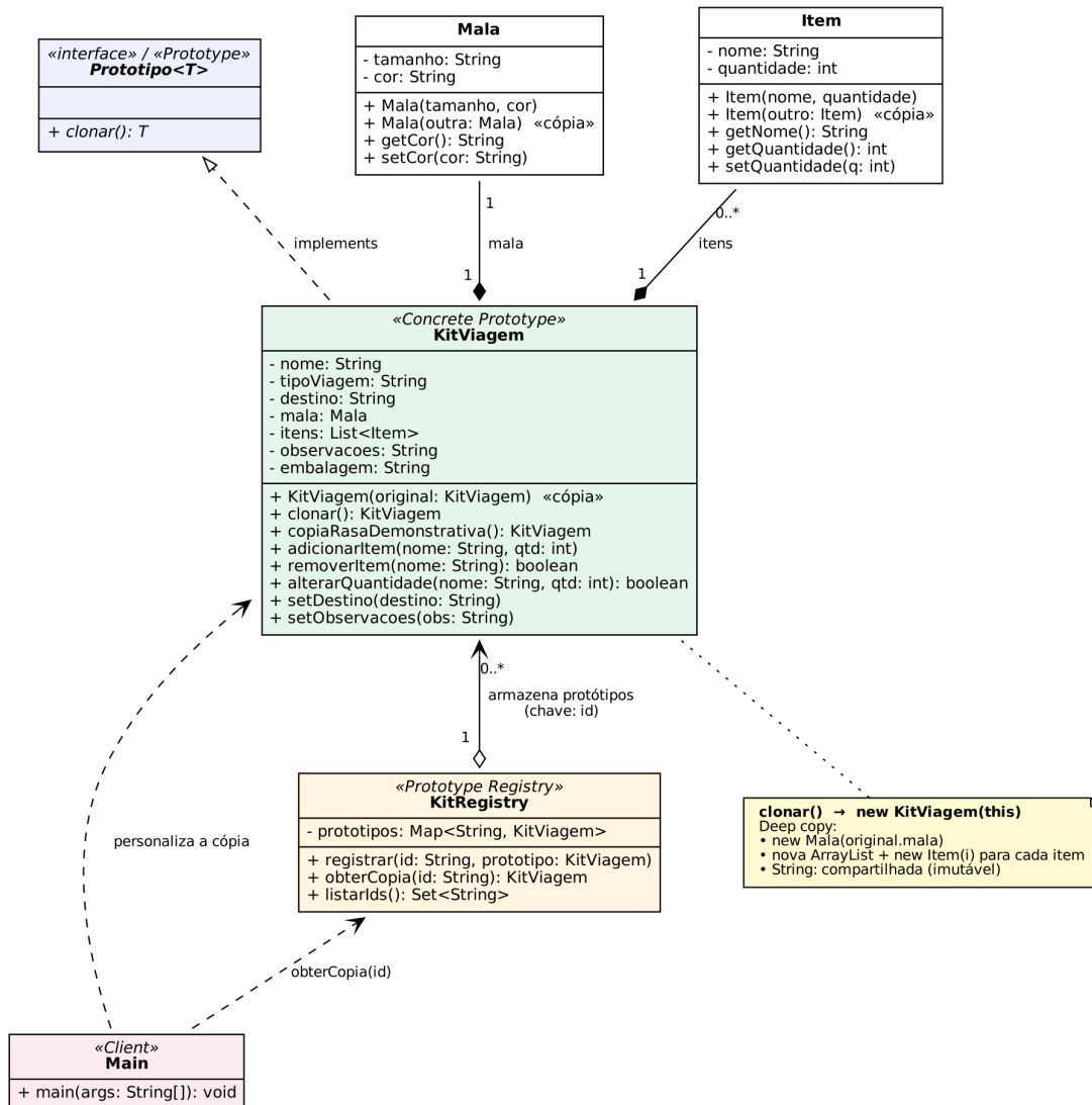
Diagrama de Classes UML — Kits de Viagem (Padrão Prototype)
