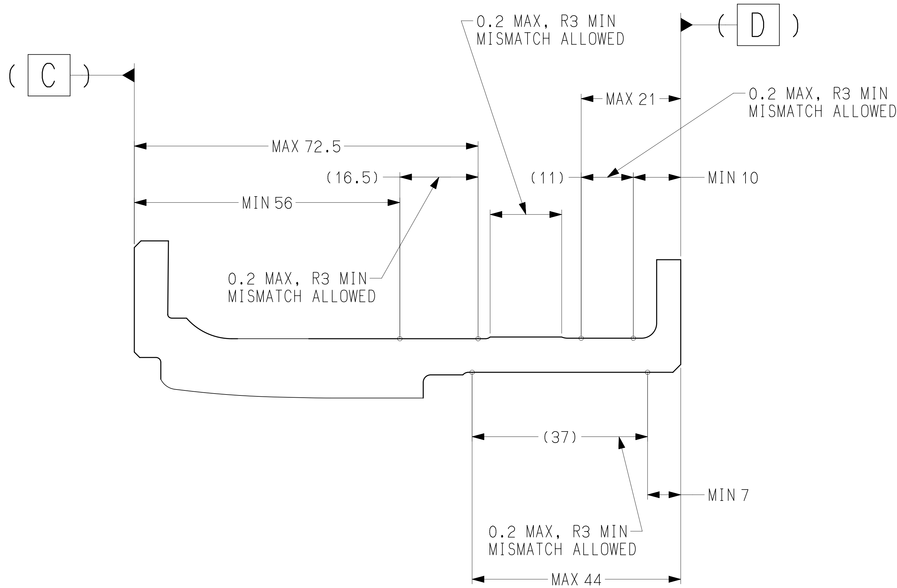
SECTION JA-JA (K3-9)
