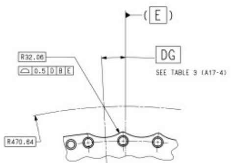
DETAIL DH (D6-4) SCALE 1:1 58 PLACES
