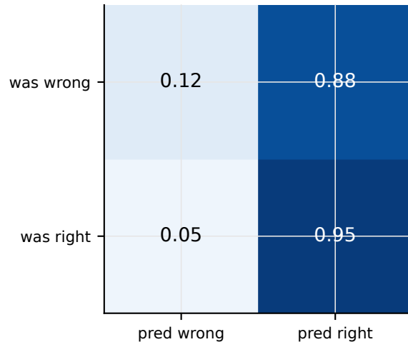
ednet_kt1 lightgbm
