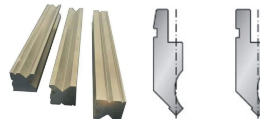
PUNCH & DIE
