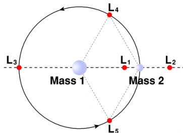
Figura: Gràfic del PRCP3C amb els punts de Lagrange
