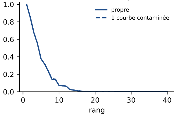
fréquence d'utilisation \hat{\phi}_j(1) , triée
