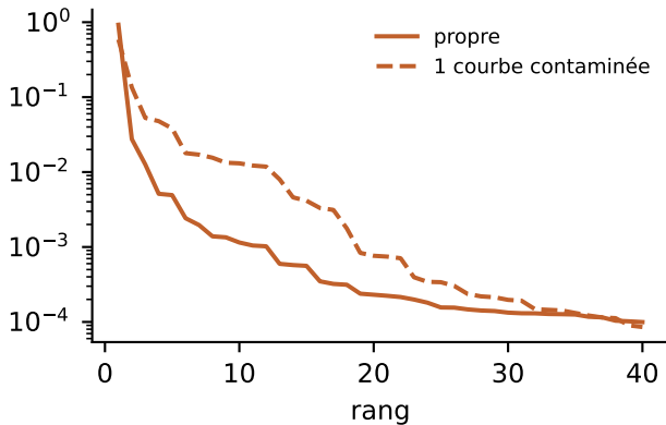
énergie (part du total), triée
