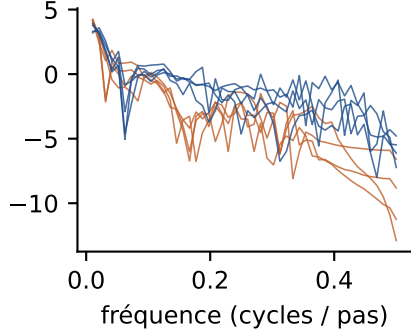
ECG200 (log-périodogramme)
