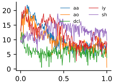
phoneme : log-périodogrammes
