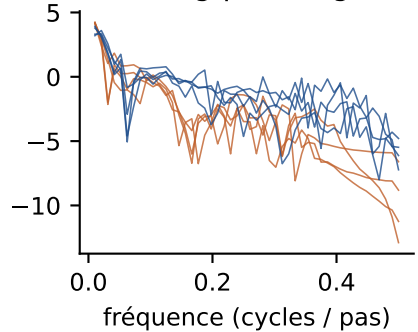
ECG200 : log-périodogrammes
