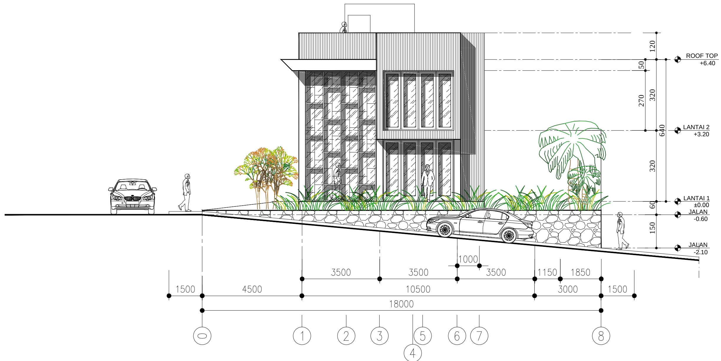
TAMPAK SP KANAN SKALA 1 : 100
