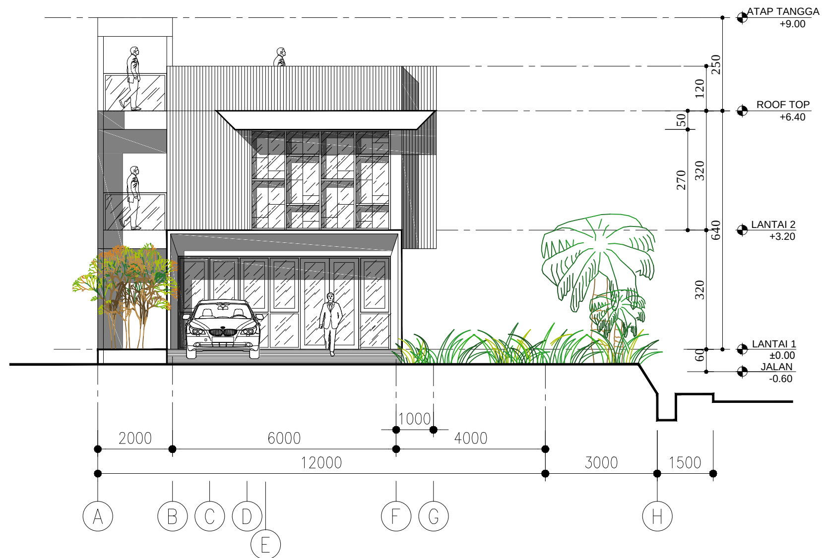
TAMPAK DEPAN SKALA 1 : 100
