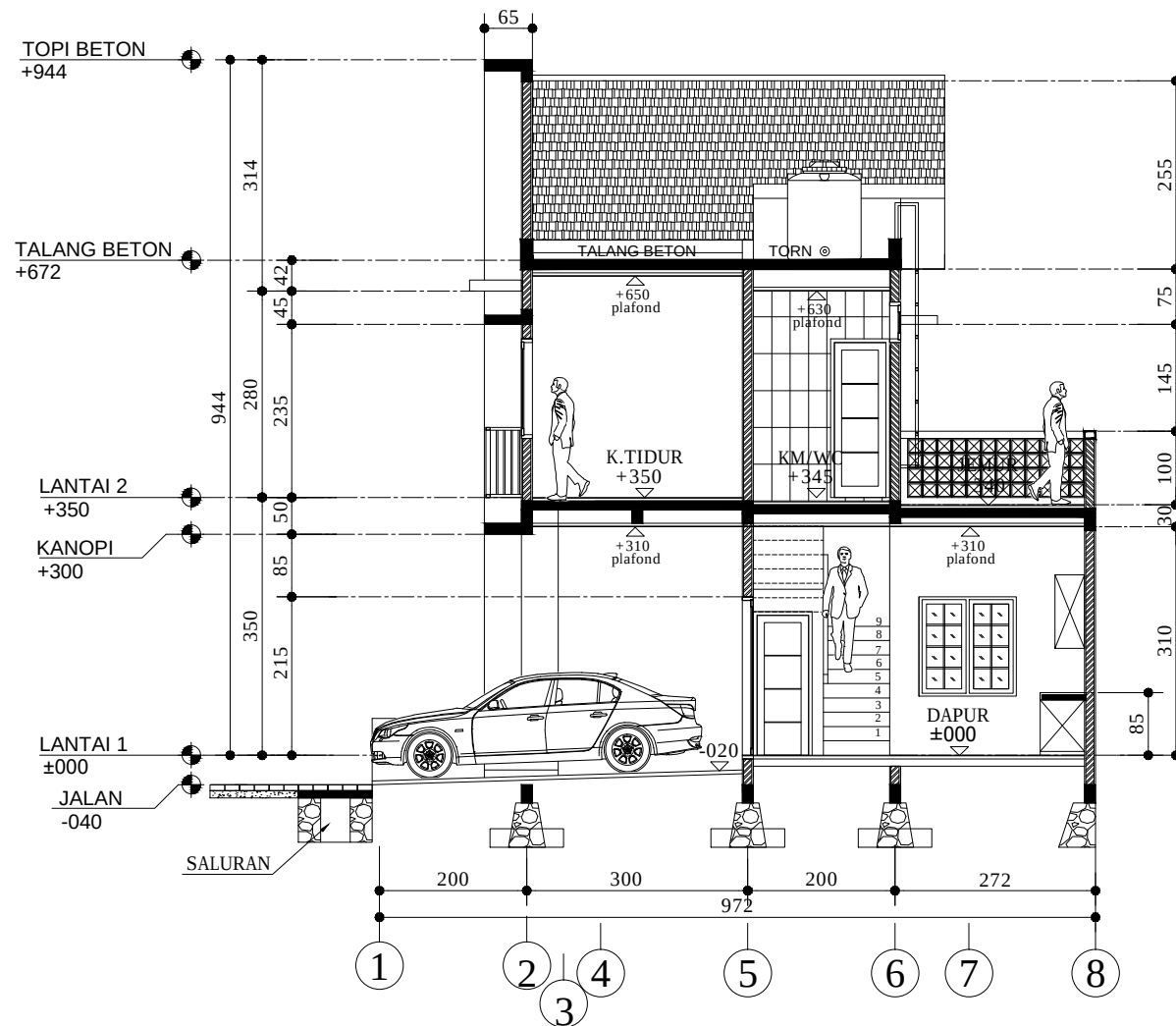
POTONGAN C-C
