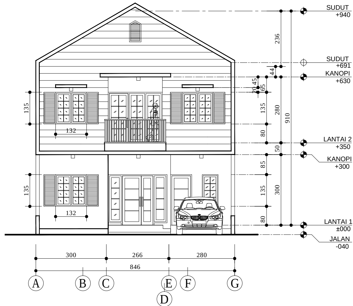
TAMPAK DEPAN SKALA 1 : 100
