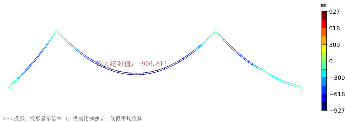
图2-16 P6 竖向位移分布
