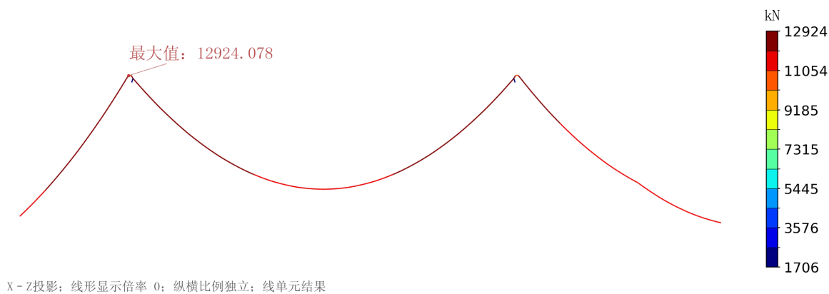
图2-17 P6 猫道承重索轴力
