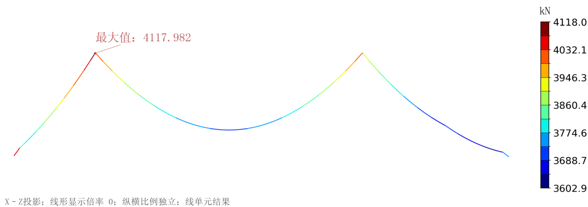
图2-18 P6 门架承重索轴力
