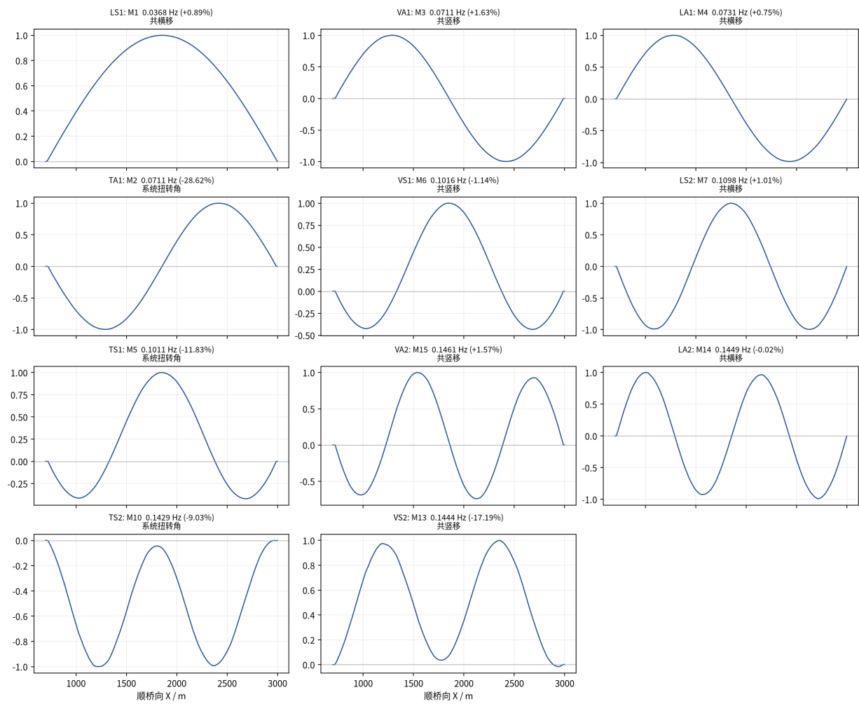
图 4: 十一个具名行配对模态的主跨观测形状 (L: 共横移; V: 共竖移; T: 系统扭转角)。
