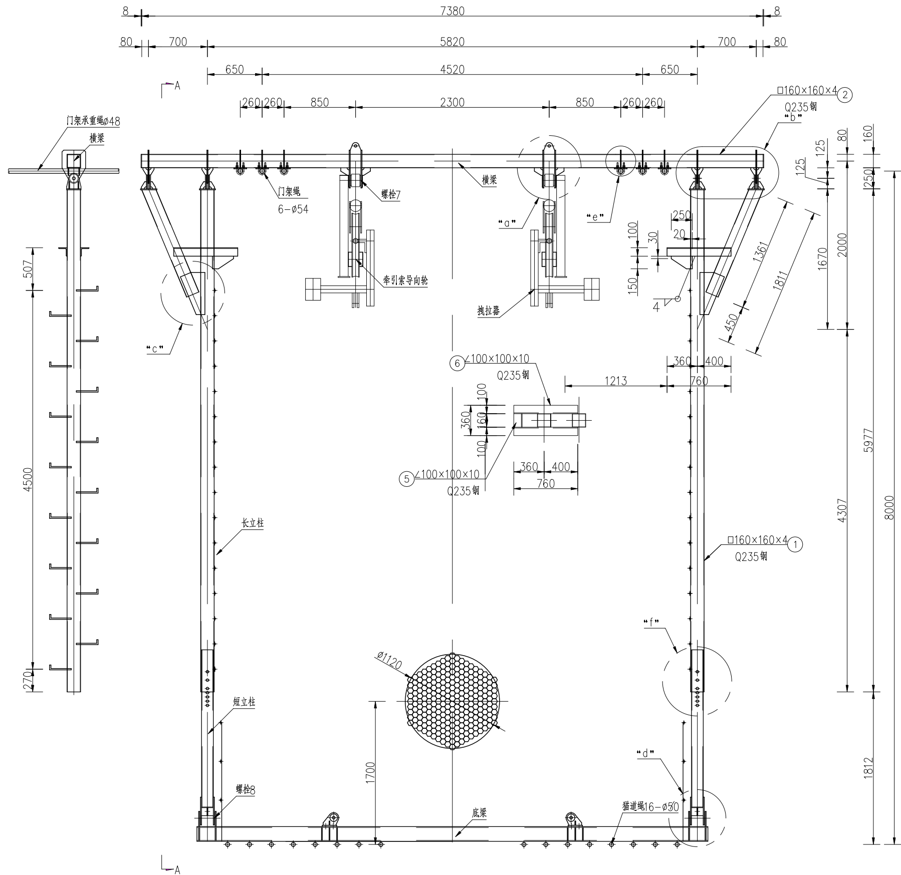
猫道门架(1)
