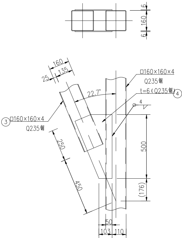
“c大样”
