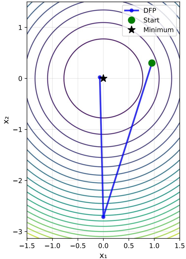
DFP Trajectory (lambda=0.1)
