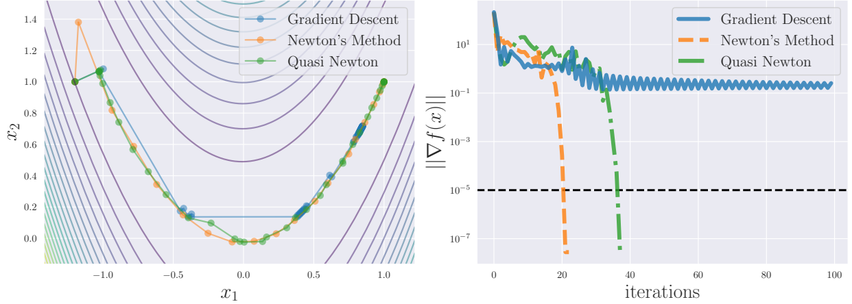
Figure 6: ニュートン法、準ニュートン法、勾配降下法の比較。
