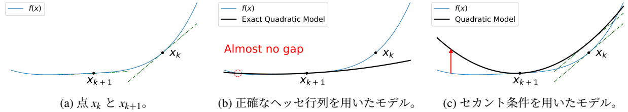
Figure 10: 標準的なセカント条件の欠点。(a) x_k と x_{k+1} での関数値と勾配が既に分かっている。(b) 正確なヘッセ行列から構築された理想的な二次モデルは、新しい点 x_{k+1} の周りでよくフィットする。(c) 標準的なセカント更新では、必ずしも十分に曲率を捉えられない。
