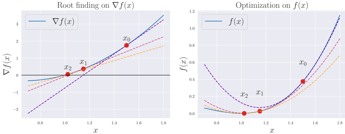
Figure 5: 勾配 \nabla f(x) = 3x^2 - 4x + 1 に対する根探索と関数 f(x) = x^3 - 2x^2 + x に対する最適化。
