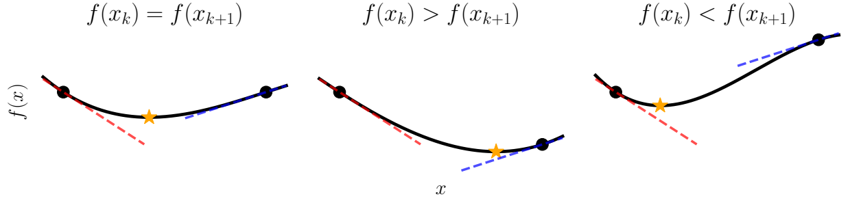
Figure 11: x_k と x_{k+1} で同一の勾配を持つが異なる関数値による内挿。これは異なる内挿関数を生じさせ、ヘッセ行列の近似に関数値情報を組み込むことの重要性を強調しています。
