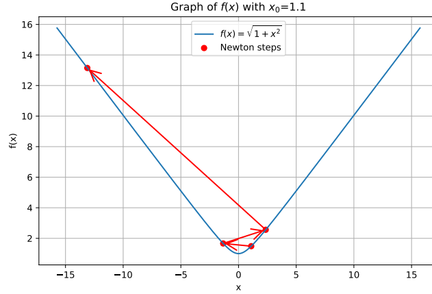
Figure 3: 初期点 x_0 = 1.1 でニュートン法が発散する例
