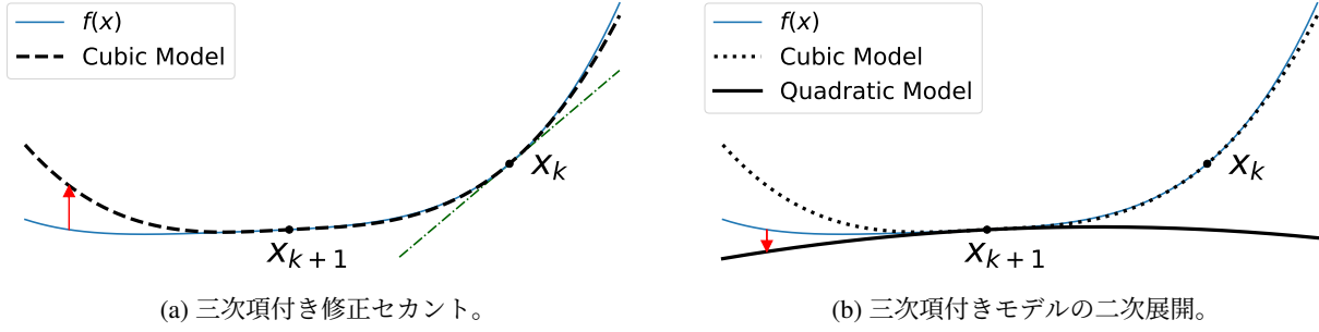
Figure 13: 三次項付き修正セカント方程式。Figure 13a では、三次項をモデルに組み込むことで、前の点で関数値と勾配の両方が一致します。Figure 13b では、その二次までの展開によるモデルを示しています。
