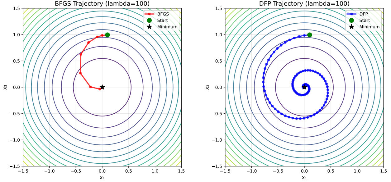
Figure 8: \lambda_1 = 100 における BFGS と DFP の反復軌跡。BFGS は 10 回で収束する一方、DFP は 107 回を要し、固有値誤差が大きい場合に BFGS が優位であることを示しています。
