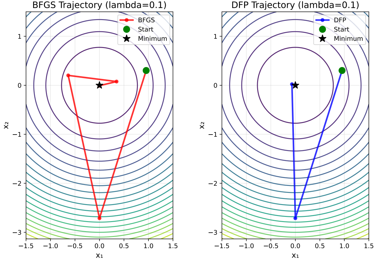
Figure 9: \lambda_1 = 0.1 における BFGS と DFP の反復軌跡。どちらも素早く収束し、DFP が BFGS よりわずかに速くなっています。
