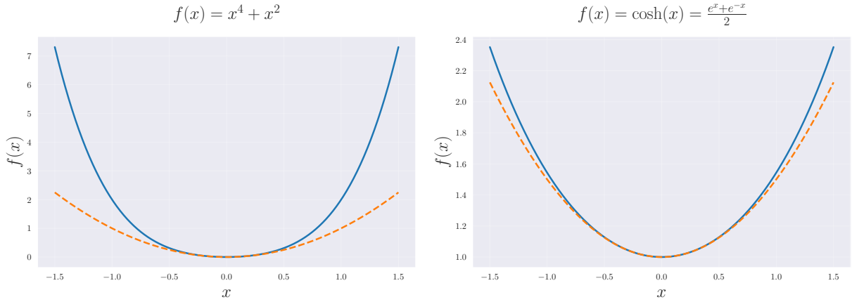
Figure 1: 凸関数と強凸関数の例。破線は x = 0 における二次近似を示す。上 2 つの関数は凸であるが強凸でないですが、下 2 つの関数は強凸性の定義を満たす \mu > 0 が存在し、強凸となります。
