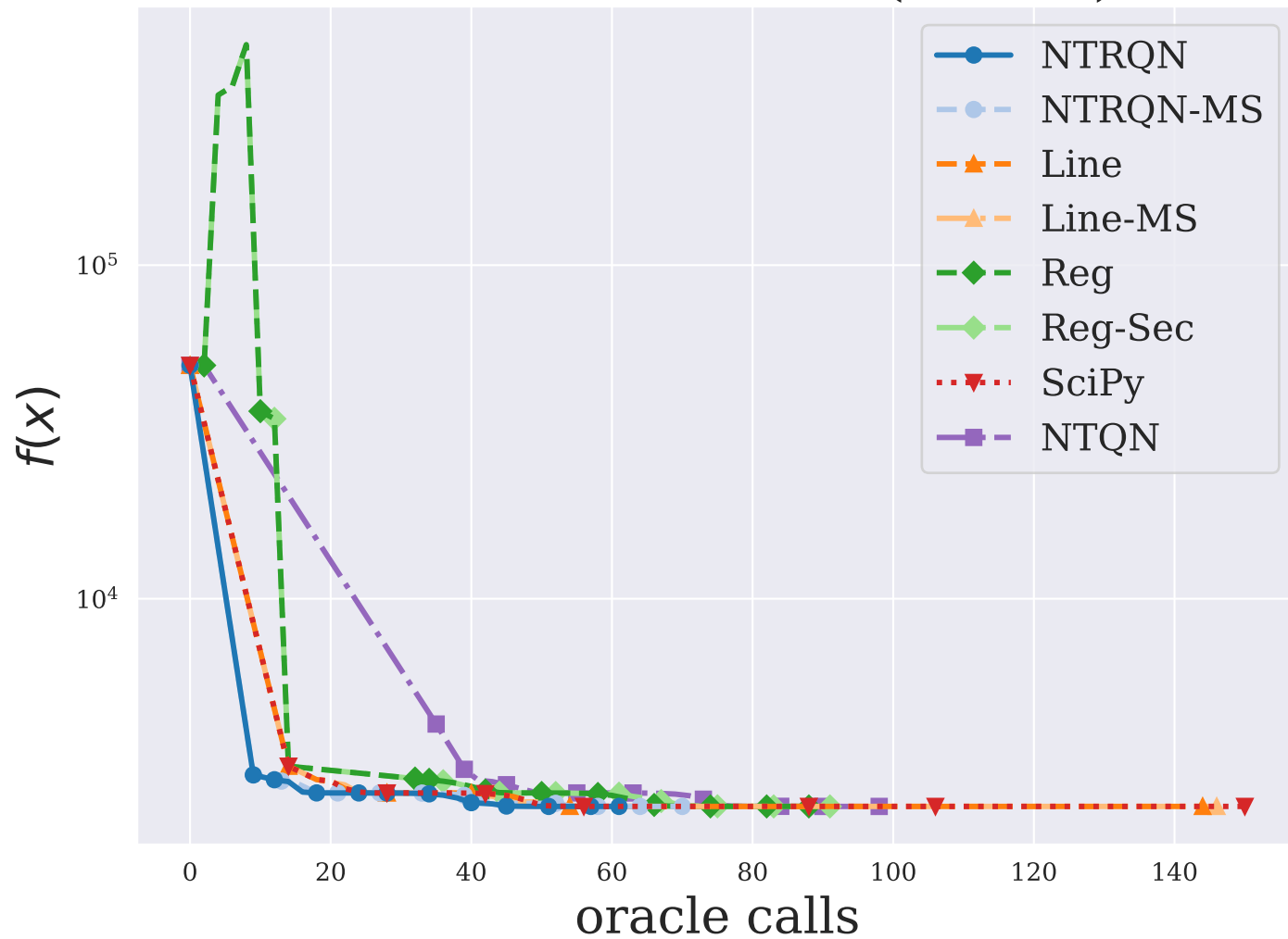
CHWIRUT1LS ( n = 3 )
