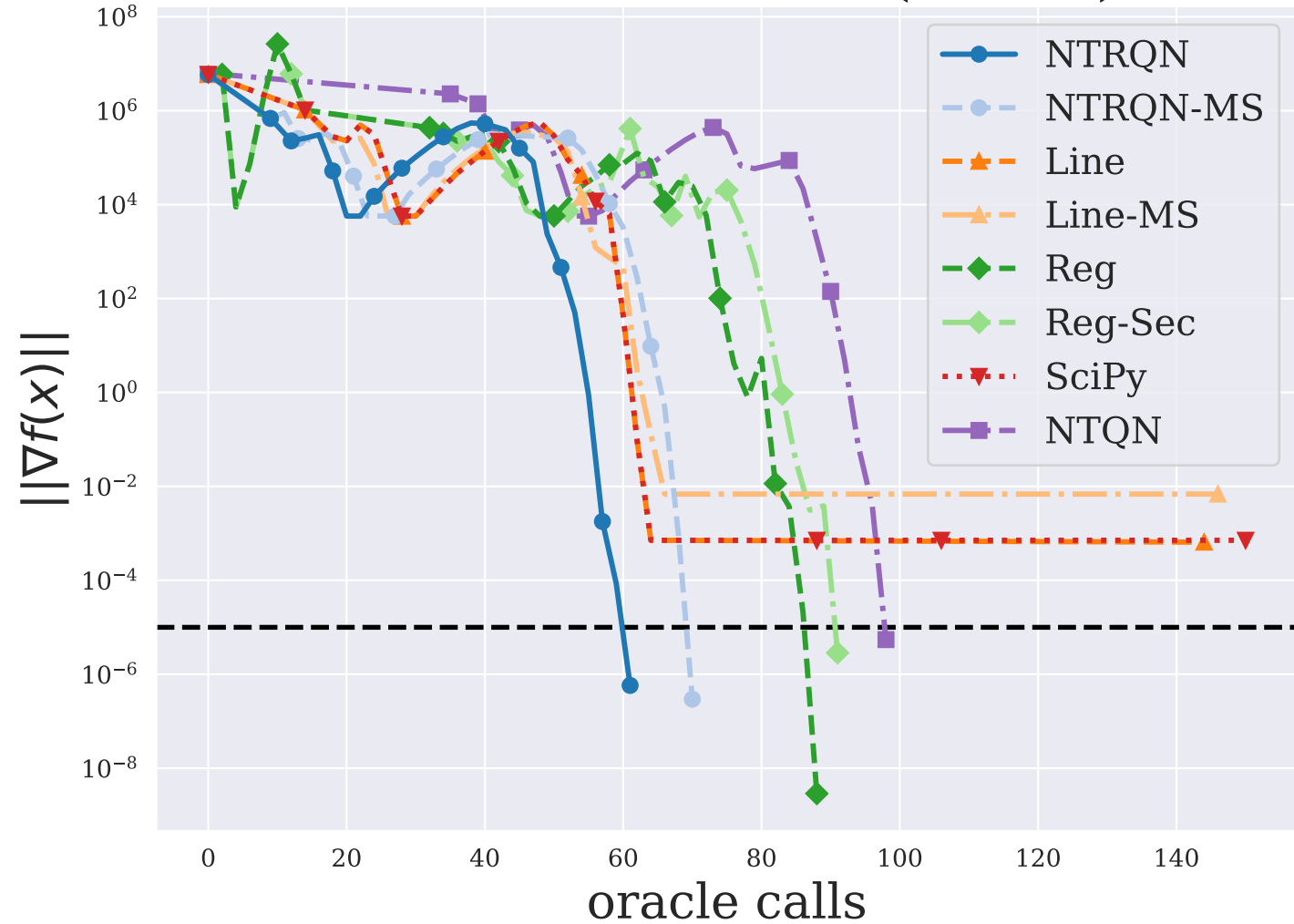
CHWIRUT1LS ( n = 3 )
