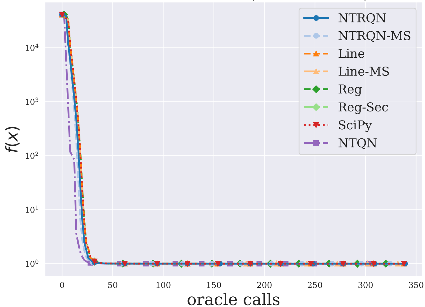
DIXMAANF ( n = 3000 )
