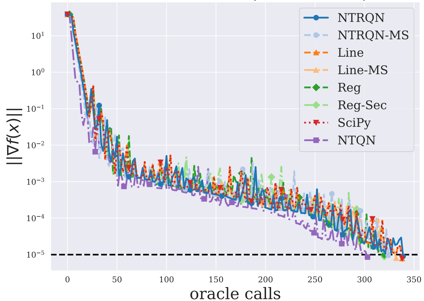
DIXMAANF ( n = 3000 )
