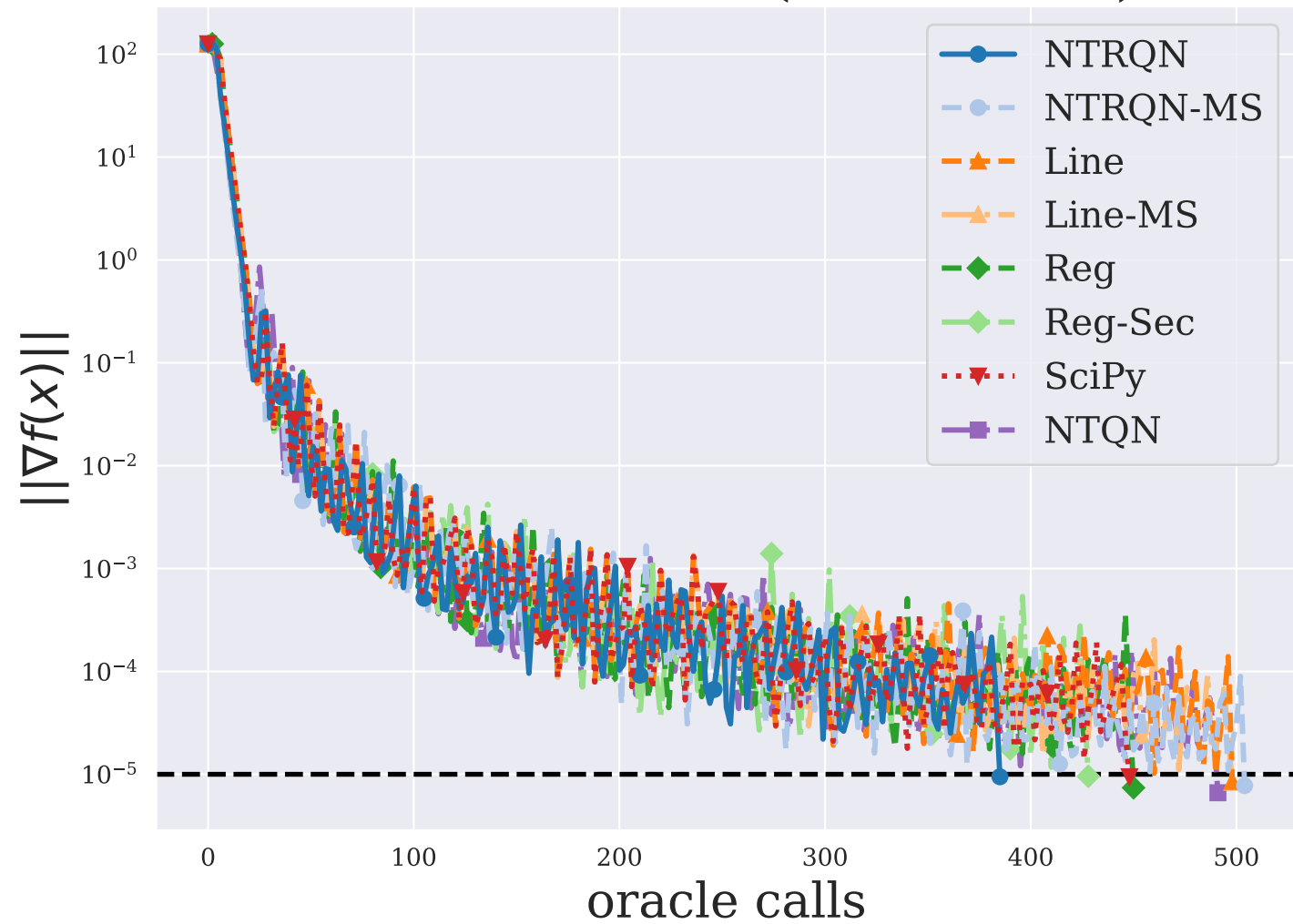
DIXMAANP ( n = 3000 )
