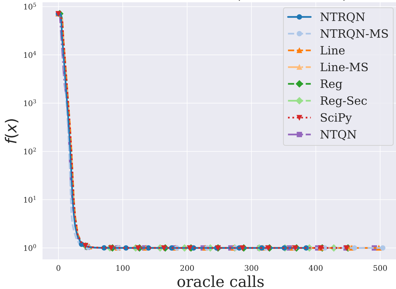
DIXMAANP ( n = 3000 )
