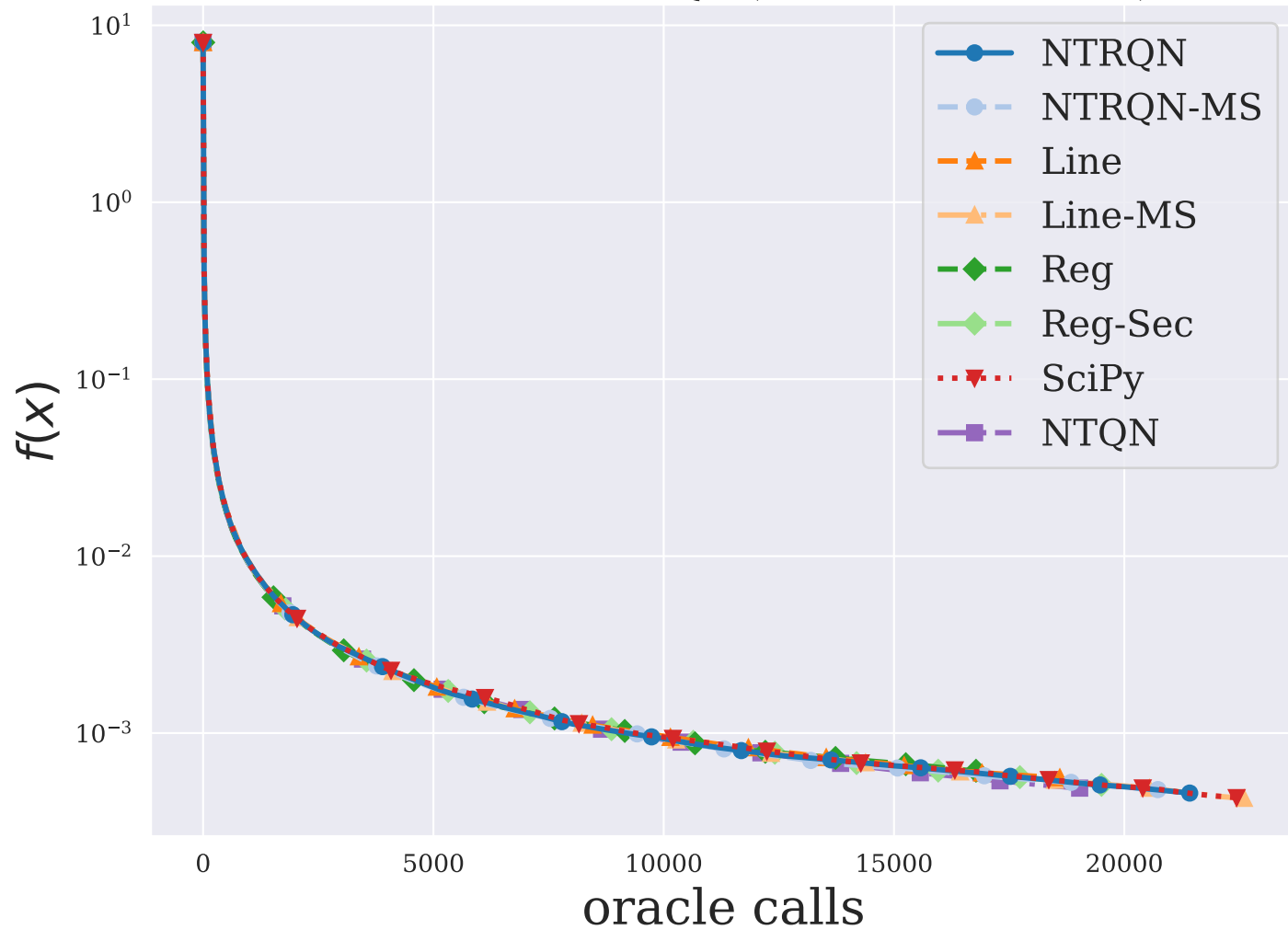
DIXON3DQ ( n = 10000 )
