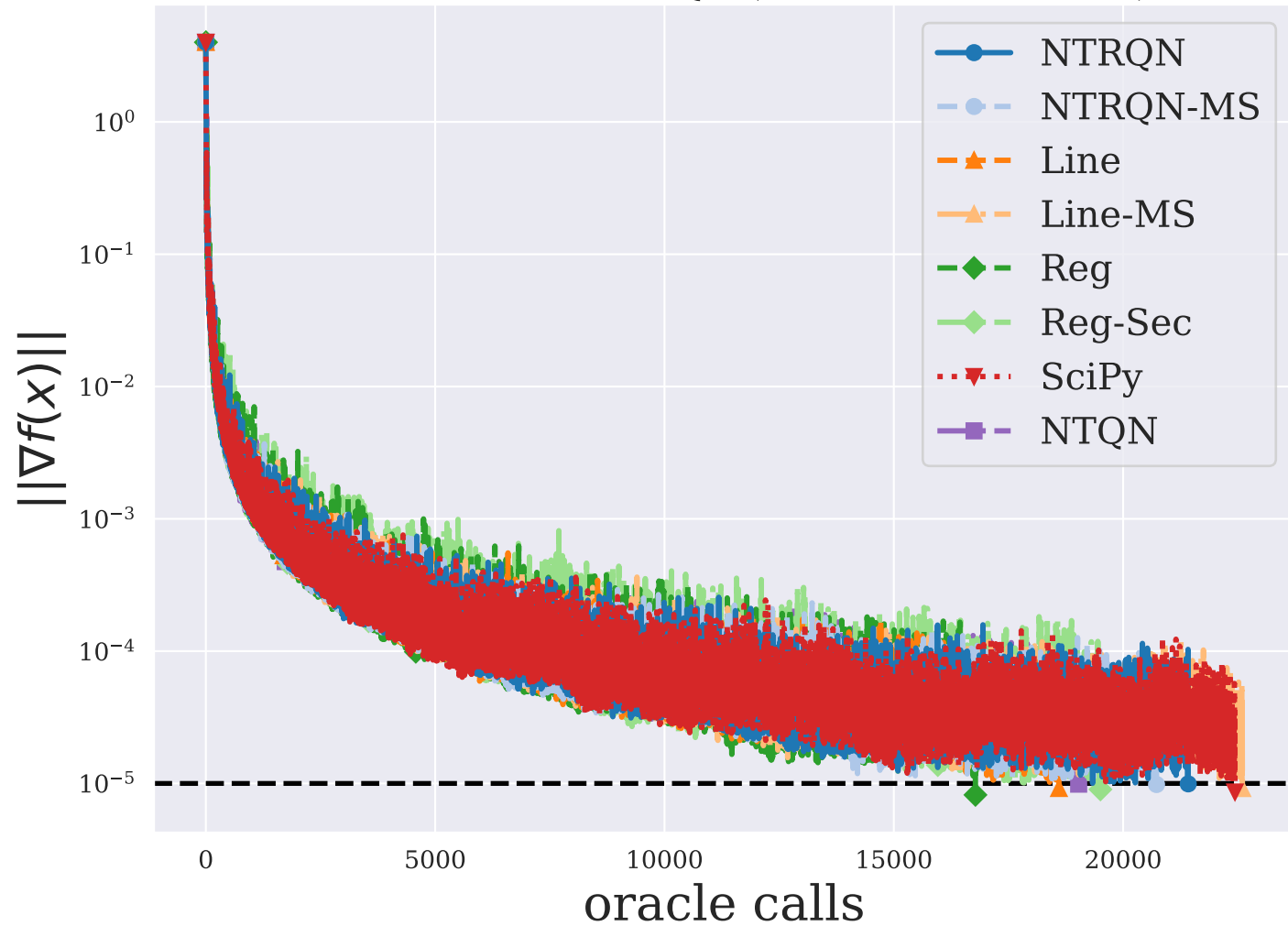
DIXON3DQ ( n = 10000 )
