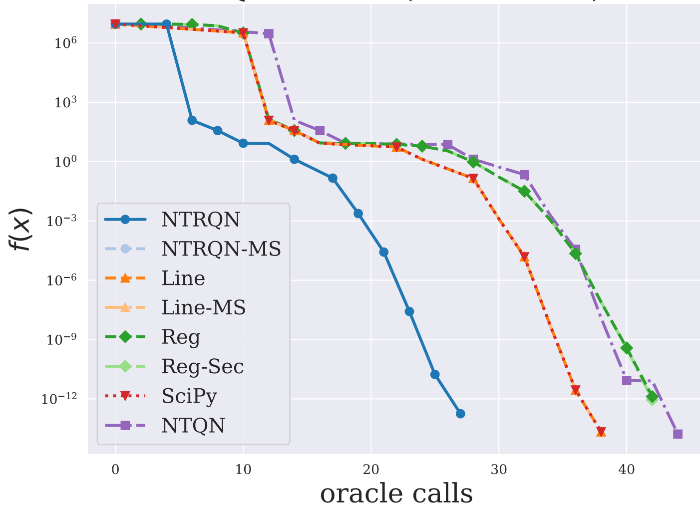
DQDRTIC ( n = 5000 )
