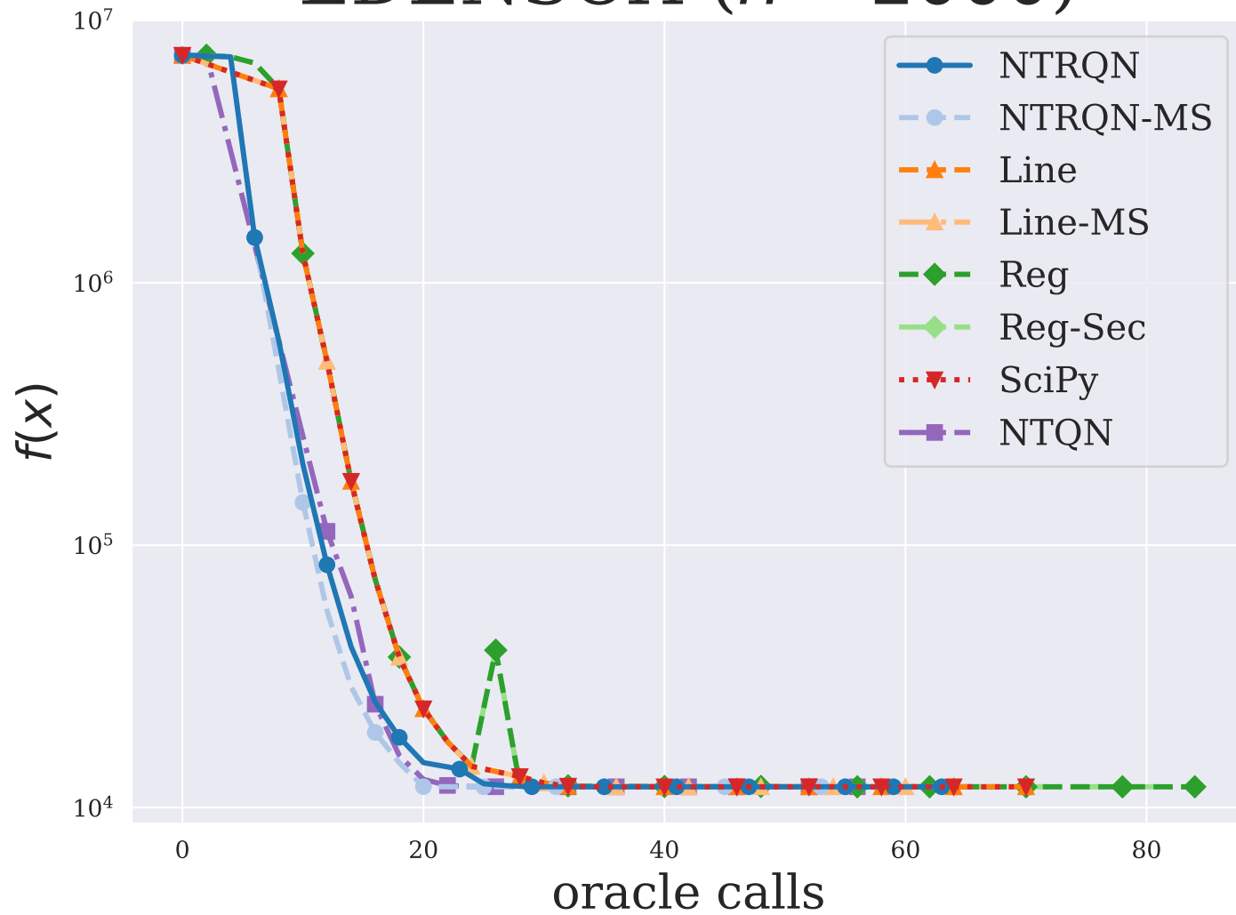
EDENSCH ( n = 2000 )
