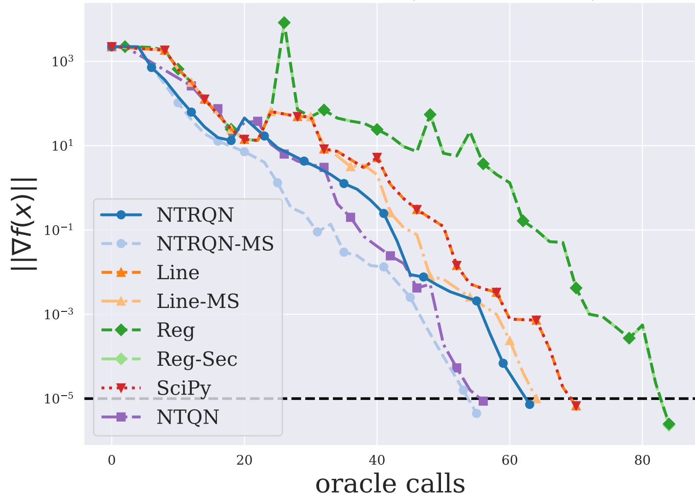
EDENSCH ( n = 2000 )
