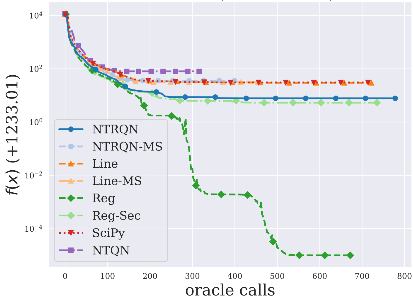
NCB20 ( n = 5010 )
