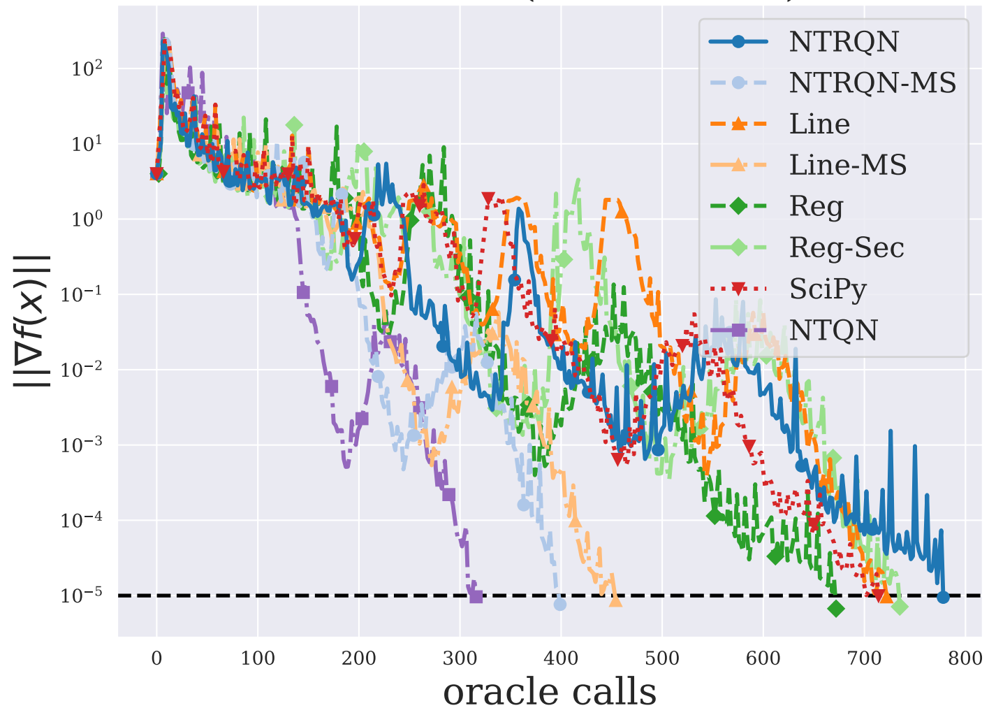
NCB20 ( n = 5010 )
