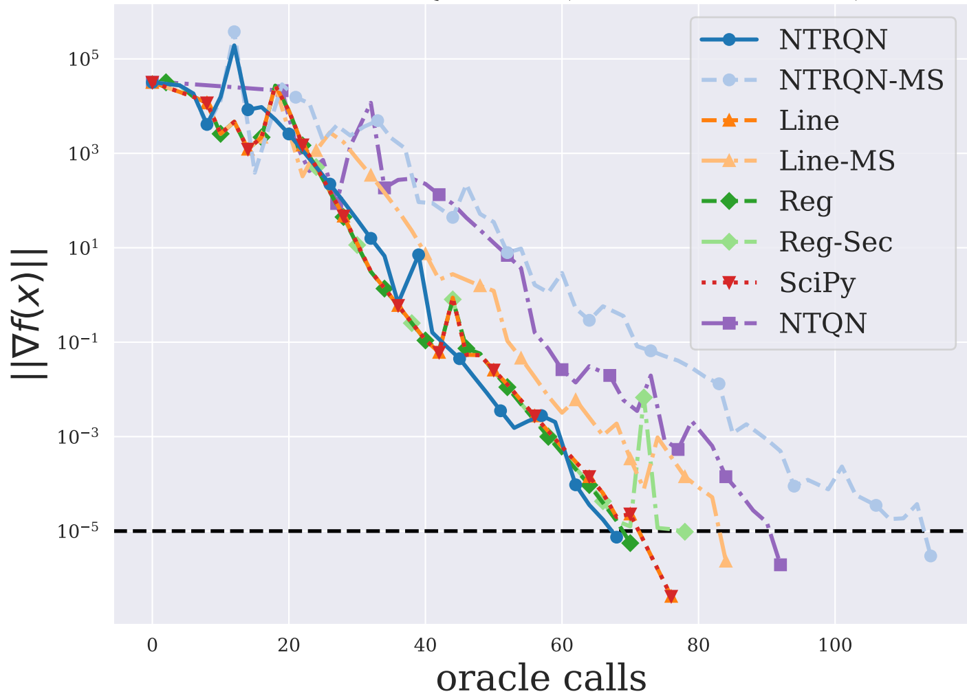
SPARSQUR ( n = 10000 )
