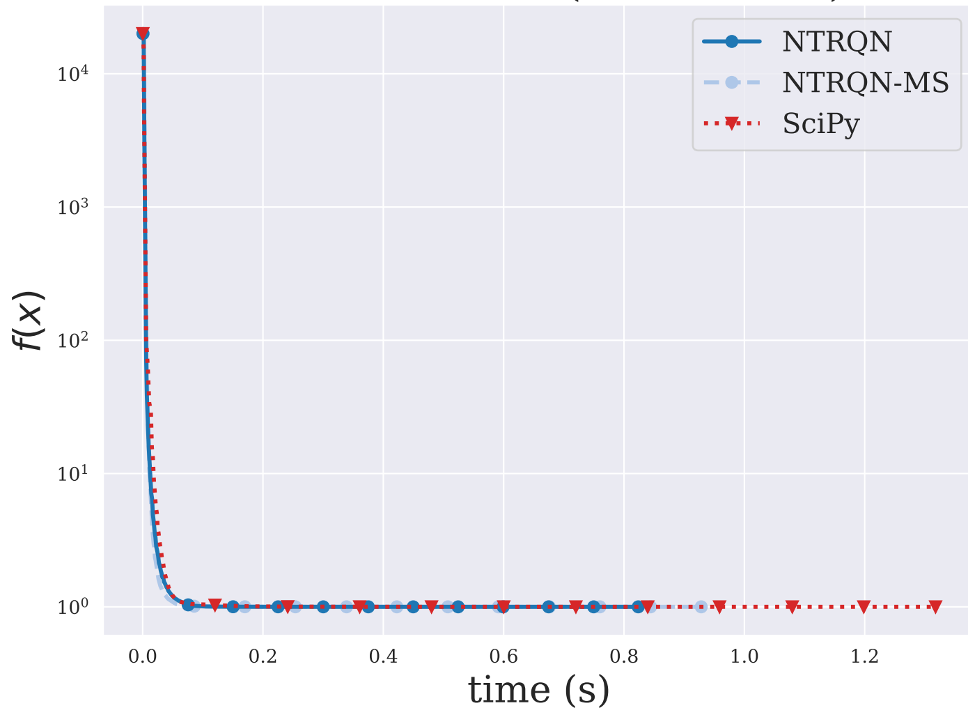
DIXMAANI ( n = 3000 )
