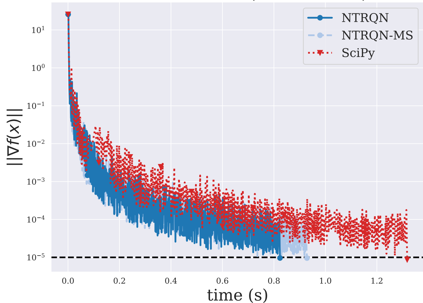
DIXMAANI ( n = 3000 )
