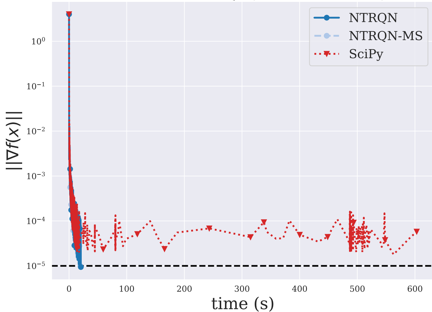
DIXON3DQ ( n = 10000 )
