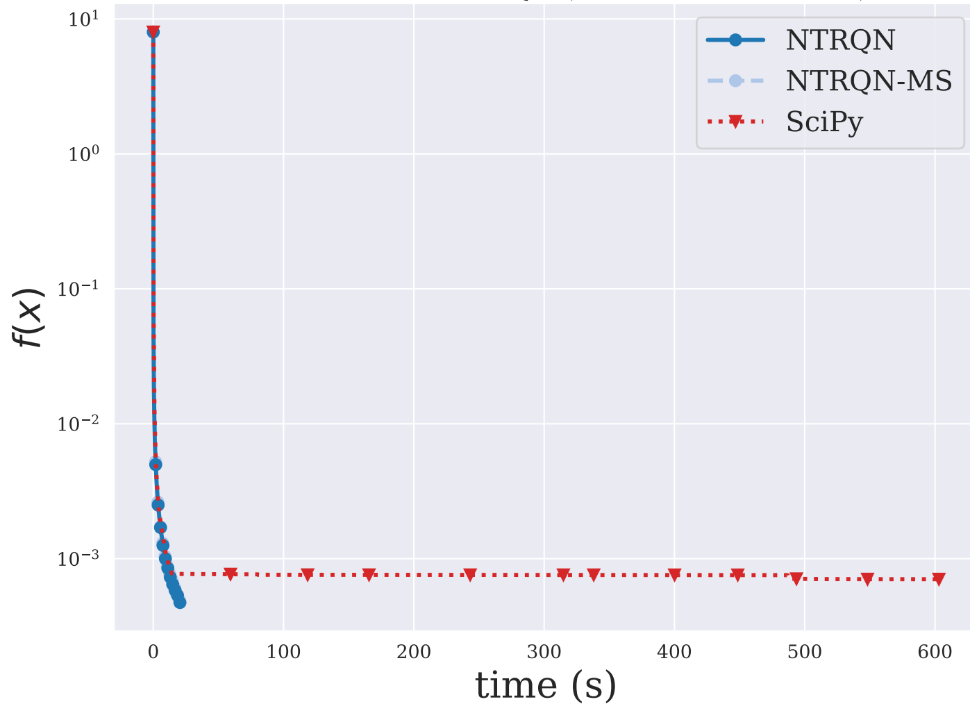
DIXON3DQ ( n = 10000 )
