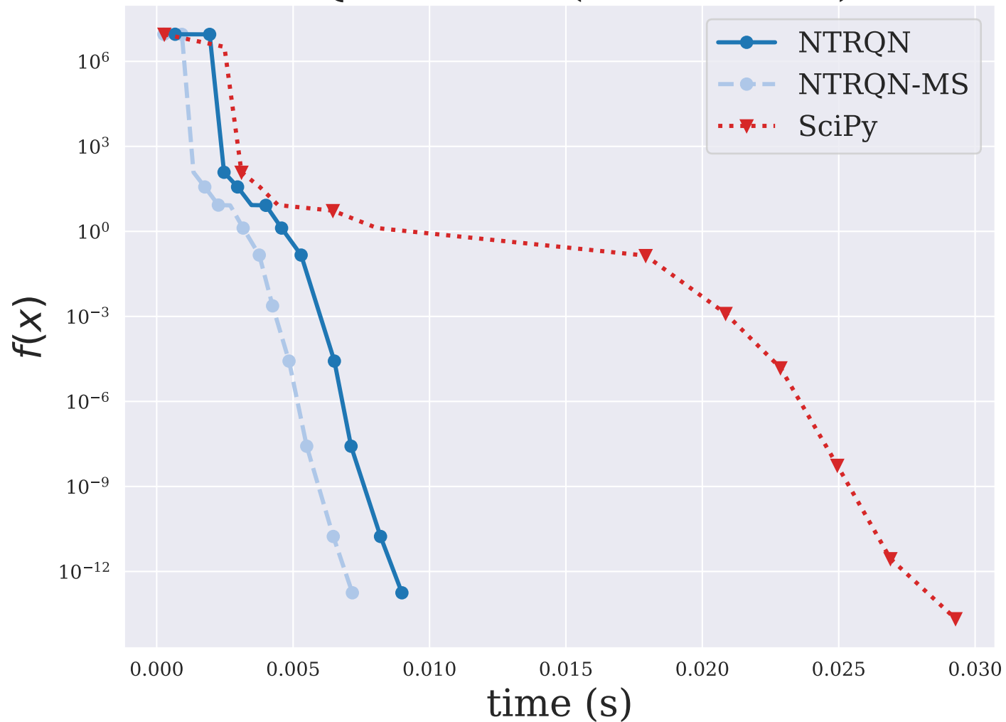
DQDRTIC ( n = 5000 )
