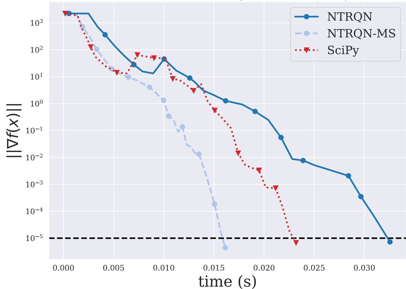
EDENSCH ( n = 2000 )
