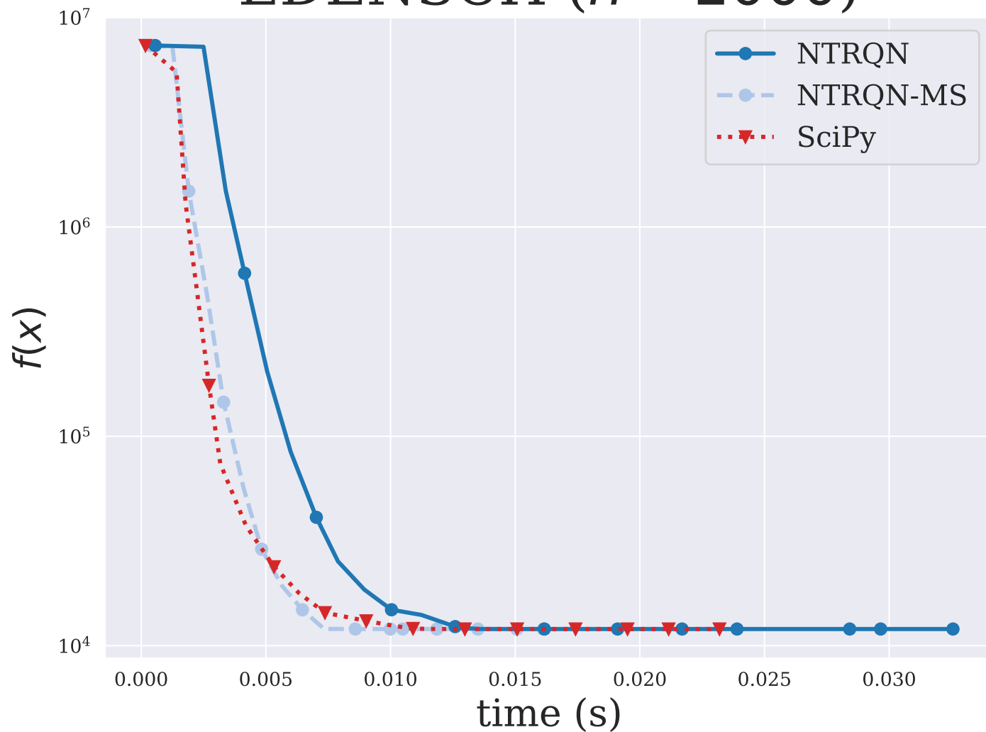
EDENSCH ( n = 2000 )
