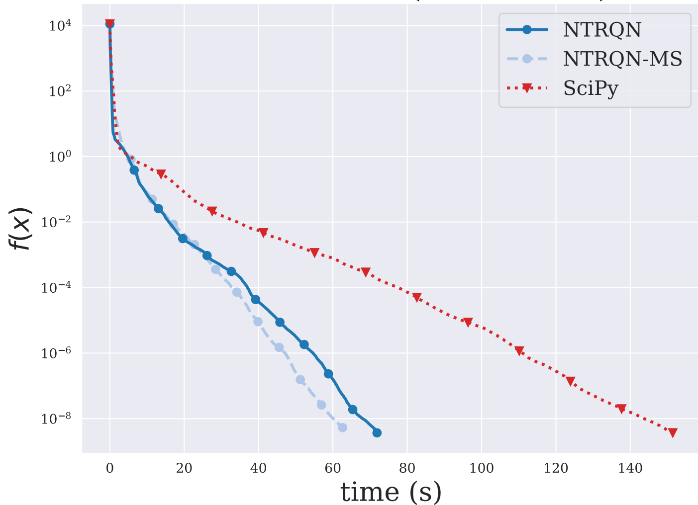
EIGENCLS ( n = 2652 )
