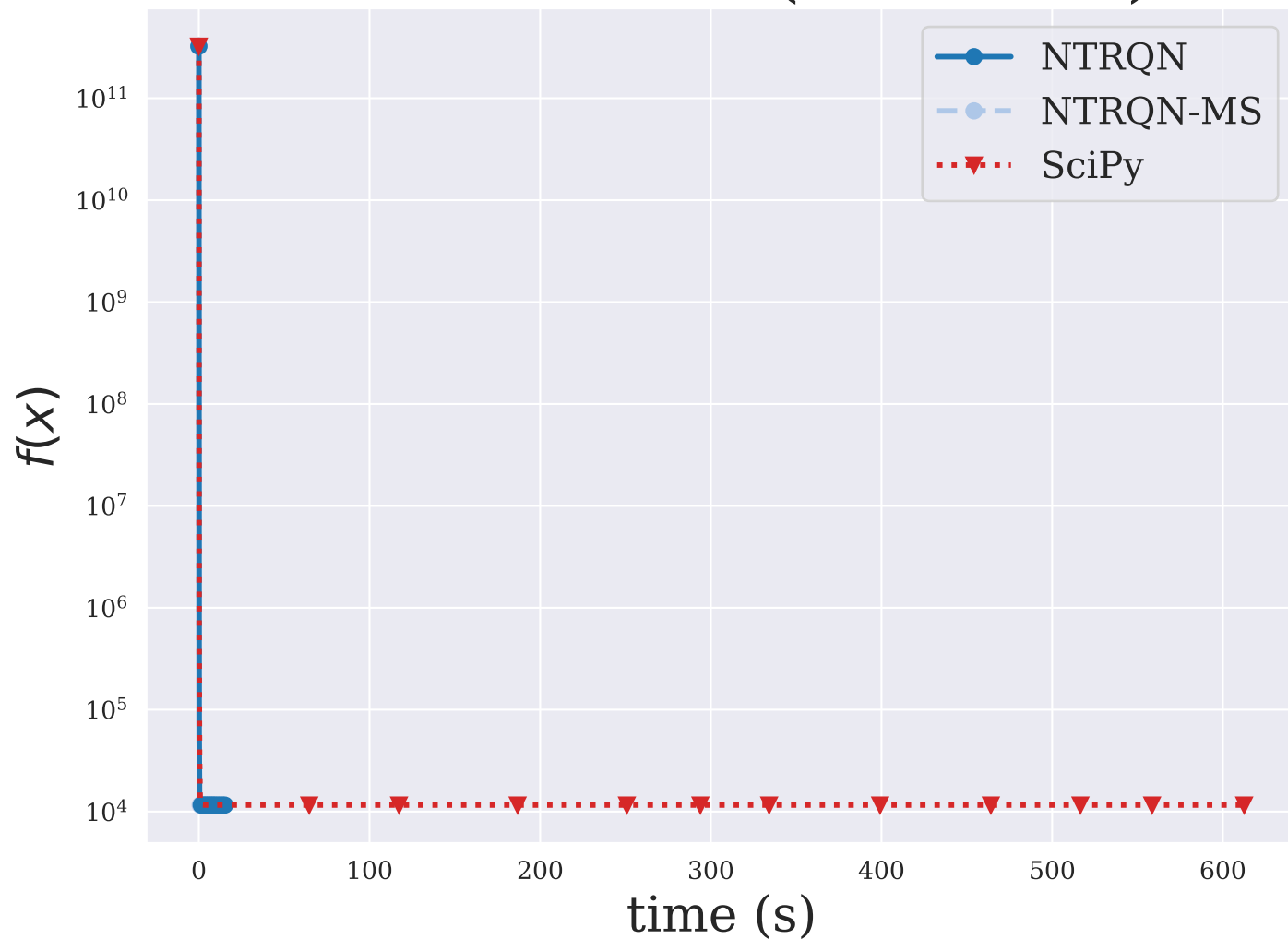
NONCVXU2 ( n = 5000 )
