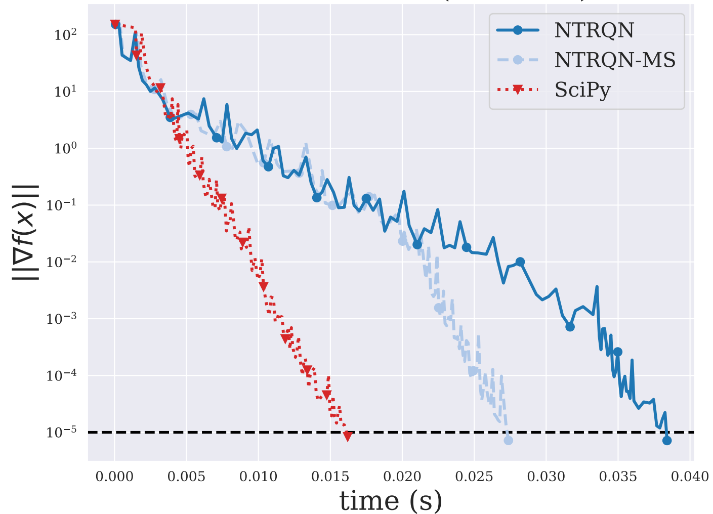
TOINTGOR ( n = 50 )
