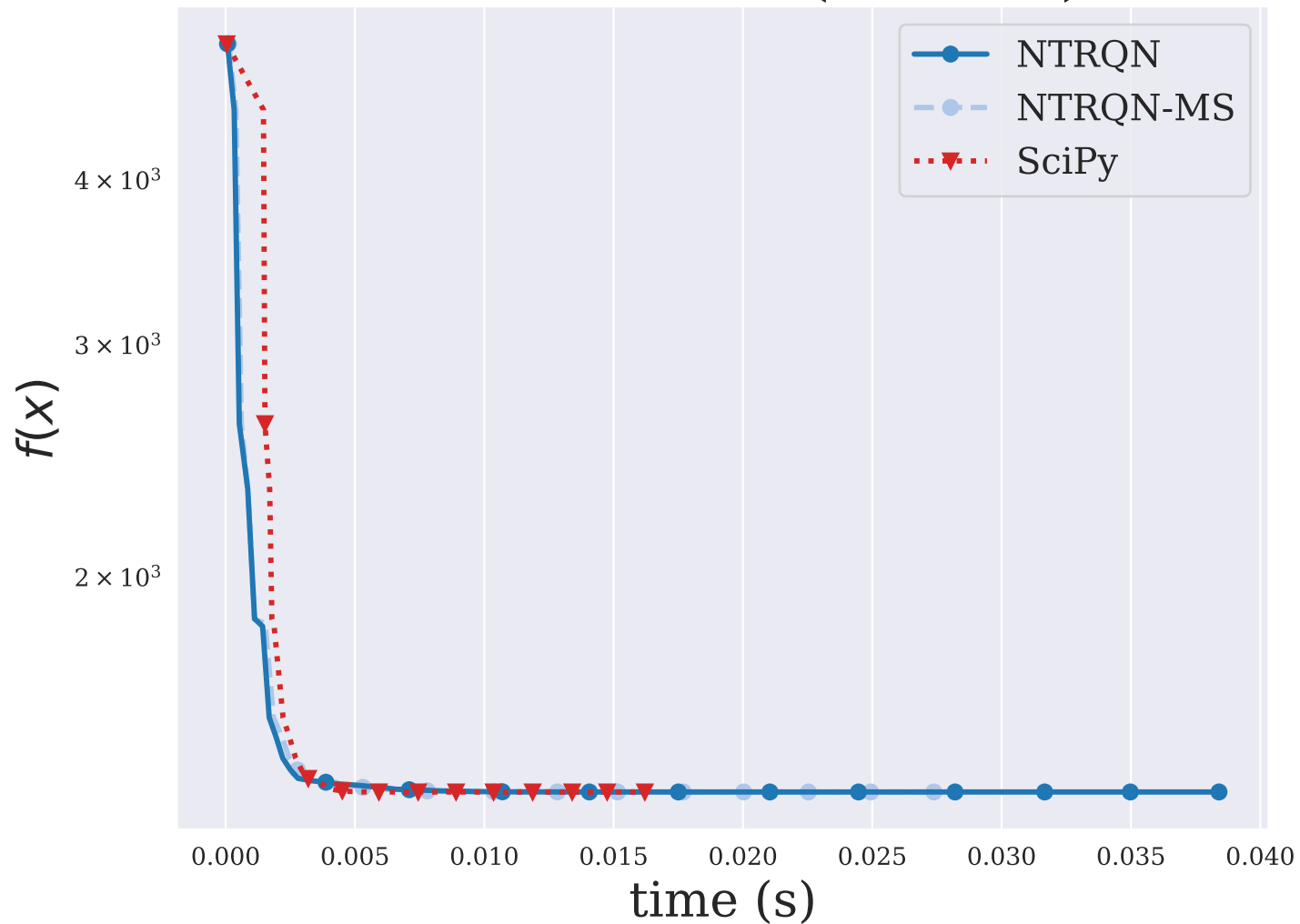
TOINTGOR ( n = 50 )
