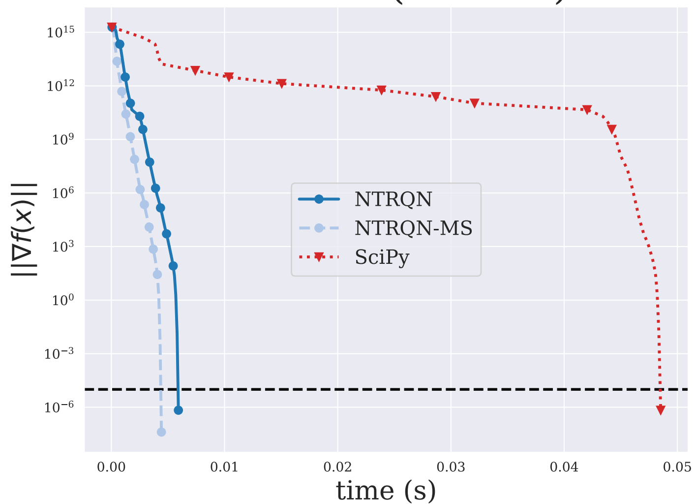
VARDIM ( n = 200 )
