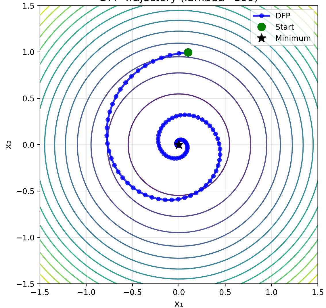
DFP Trajectory (lambda=100)
