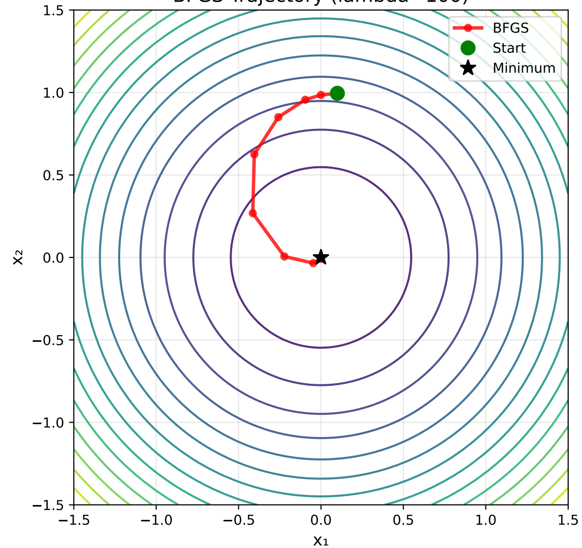
BFGS Trajectory (lambda=100)
