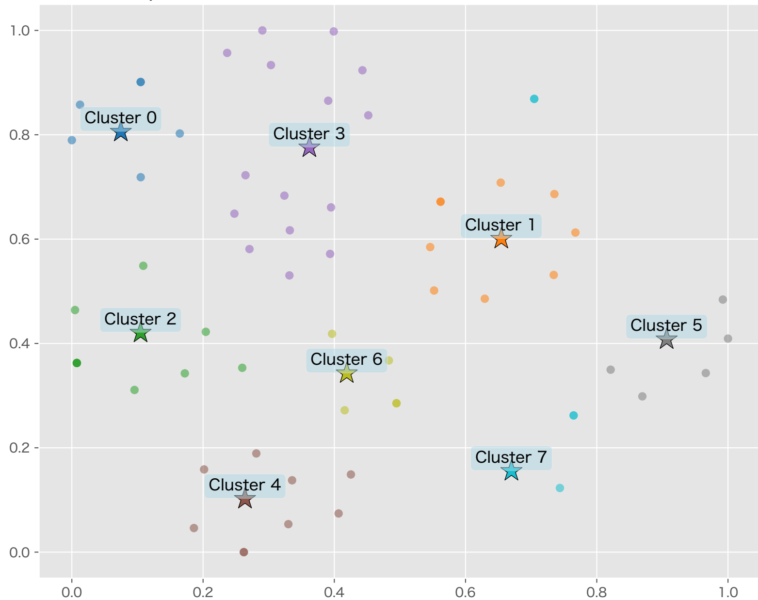
Laplacian固有空間(8次元)によるクラスタリング + t-SNE可視化
