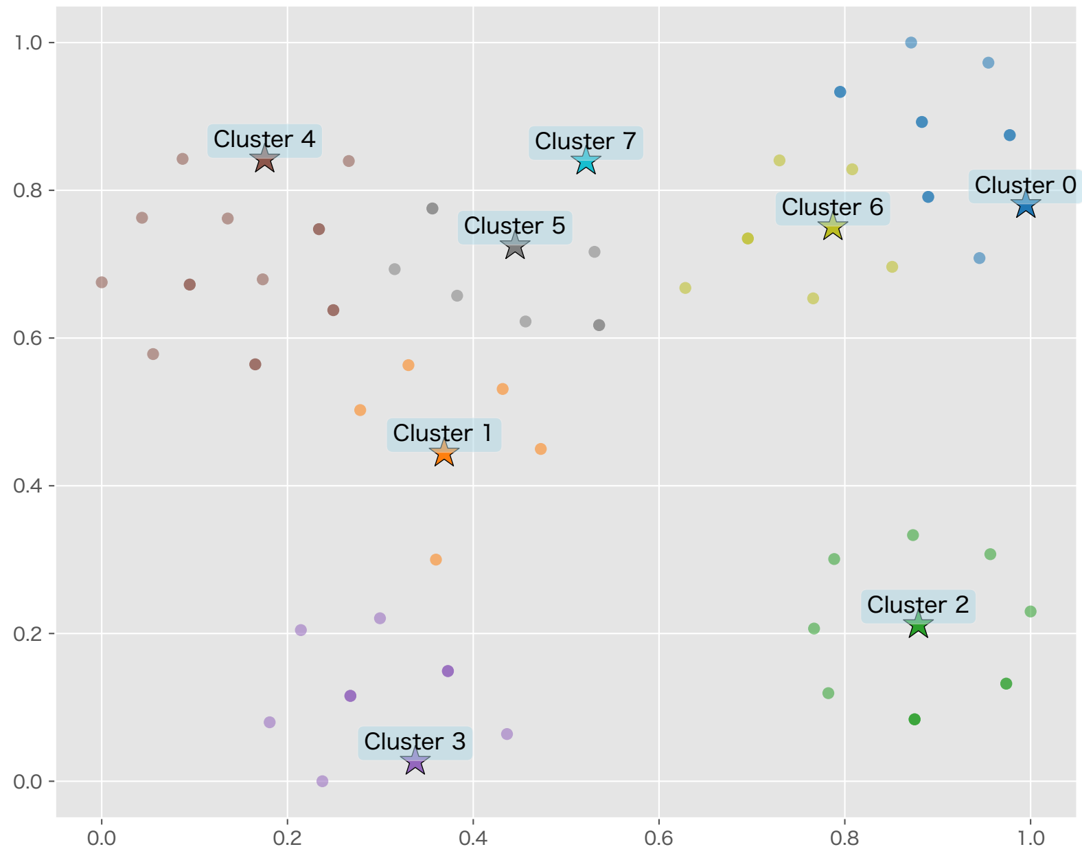
【重み付け】 Laplacian固有空間(3次元) + t-SNE可視化 (Weights: [1. 2. 1. 1.5 2. 1.5])
