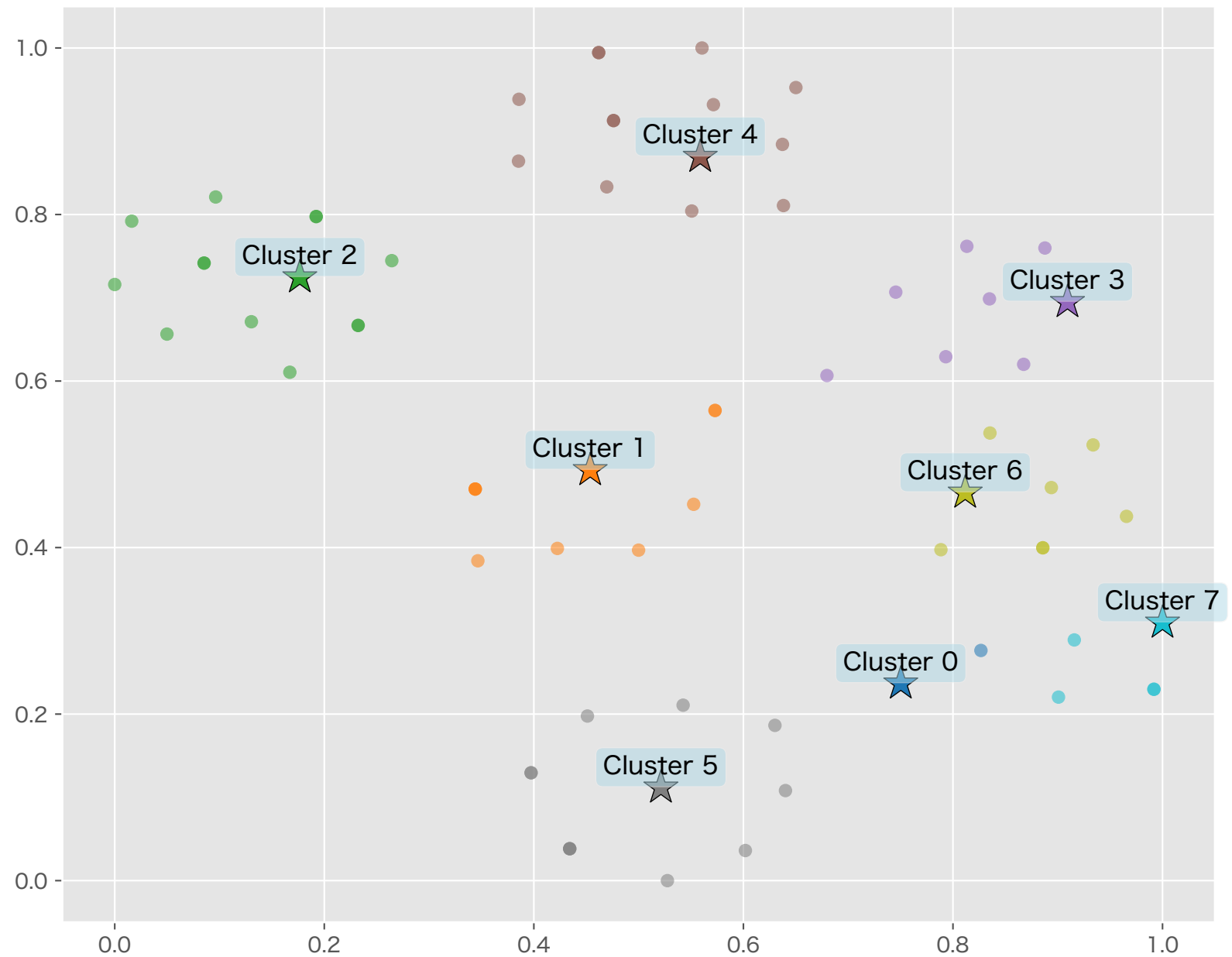
【重み付け】 Laplacian固有空間(5次元) + t-SNE可視化 (Weights: [1. 1.5 1. 1. 2. 1.])
