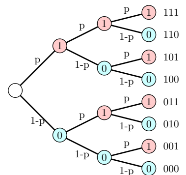
Abbildung 1.1: Bernoulli-Experiment mit drei Wiederholungen
