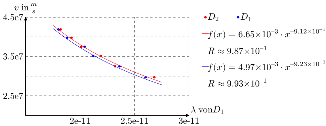
Abbildung 1.4: v - \lambda -Diagramm und Regression für die Durchmesser D_1 und D_2
