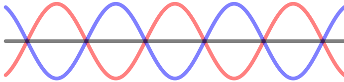
Abbildung 2: Überlagerung zwei unterschiedlicher Wellen
