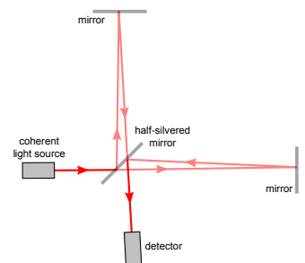
Abbildung 1: Michelson-Interferometer
