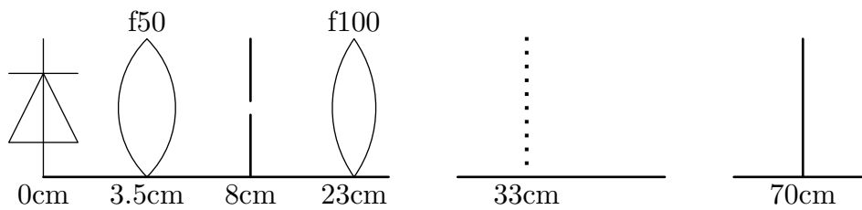
Abbildung 5.4: Aufbau
