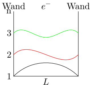
Abbildung 5.4: Modell
