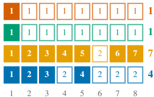
mt-illegal
