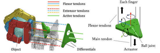
Fig.3: CS-TDM finger module
