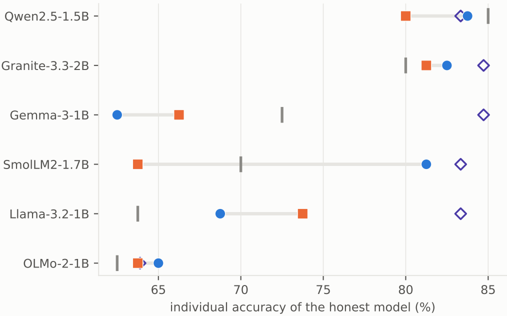
(d) H3 · BoolQ: informed – plain = +2.5 points [-1.7, +6.7]
