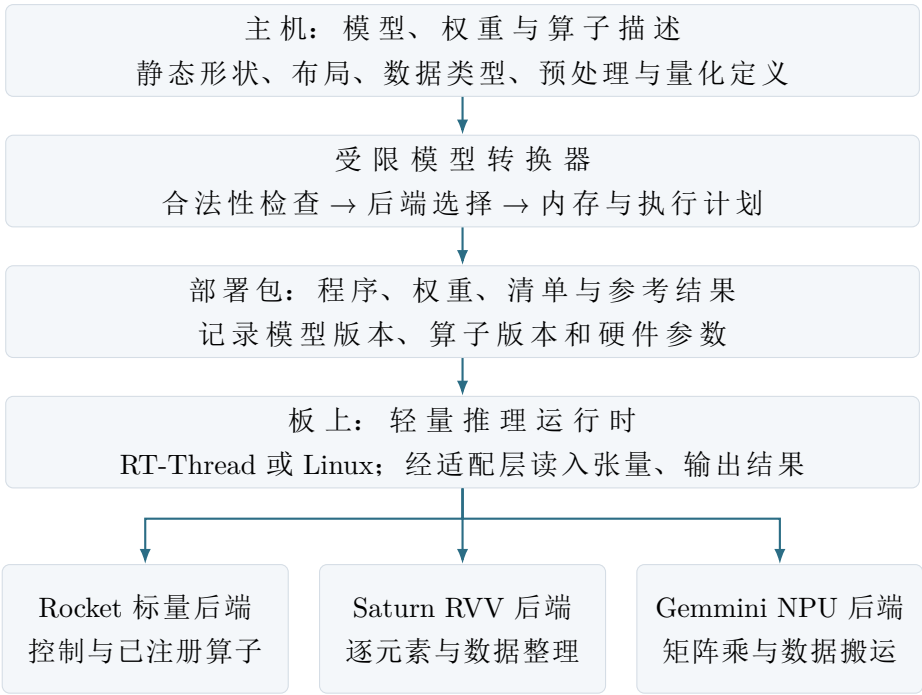
图 1 拟设计的软件体系与部署数据流
