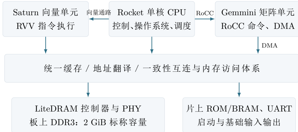
图 2 拟设计的硬件逻辑关系；地址翻译与一致性连接仍需联合适配
